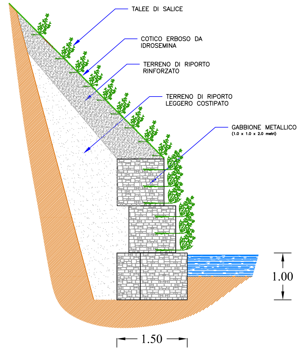
Sezione Tipo
